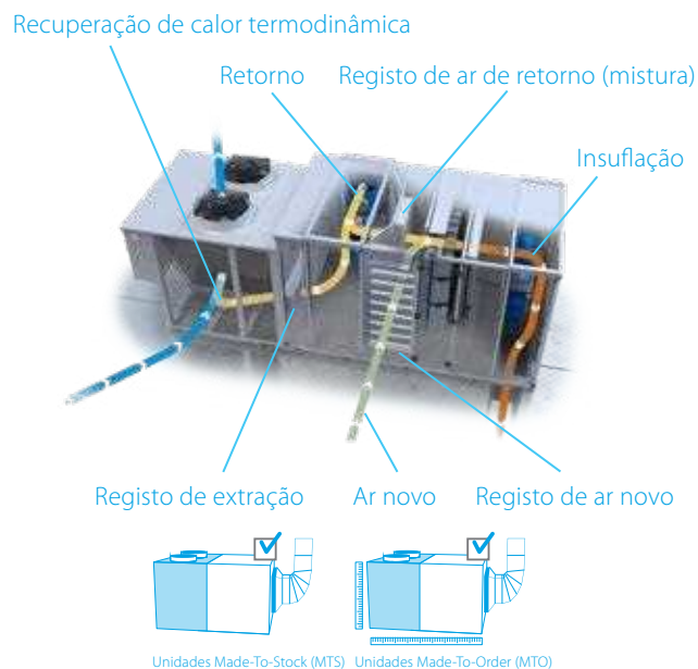
EXEMPLO DE FUNCIONAMENTO EM AQUECIMENTO
