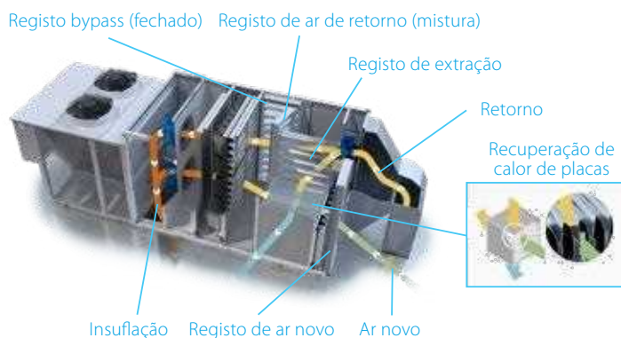
MODO DE RECUPERAÇÃO DE CALOR DE PLACAS EM OPERAÇÃO DE AQUECIMENTO
